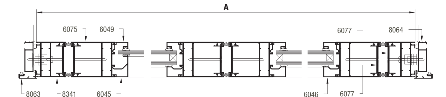
SECCION 1-6-7
